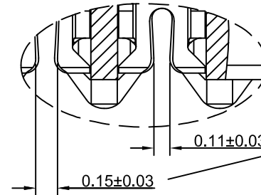
SECTION A-A SCALE 2.5:1
